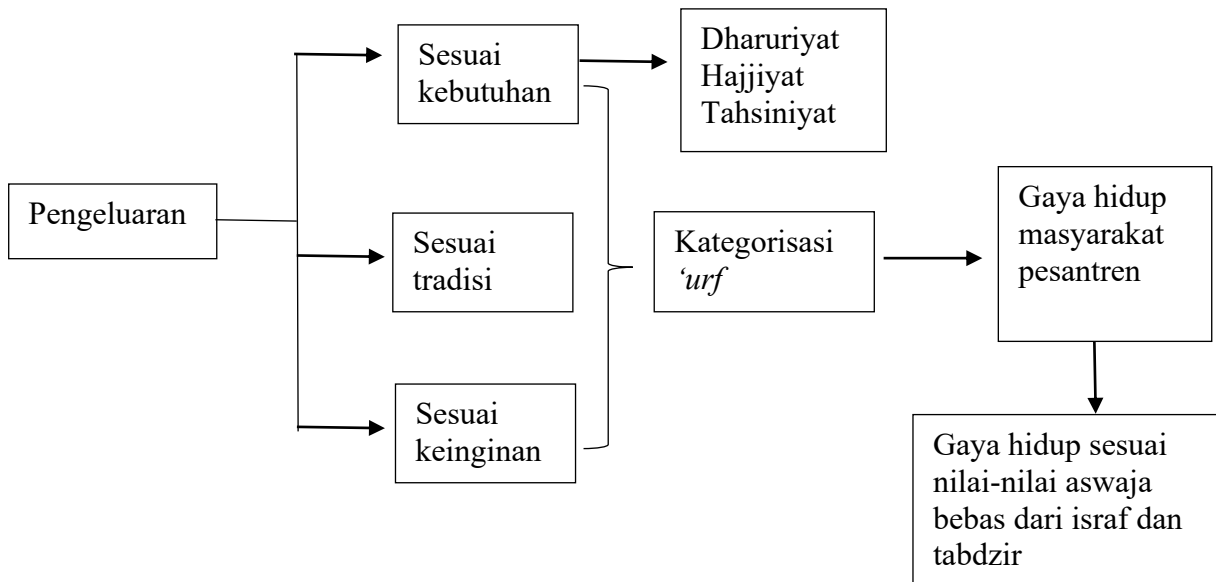
Gambar 1 kerangka penelitian
